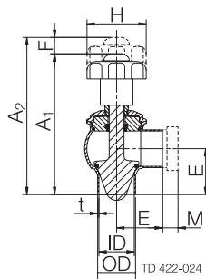
Fig. 4. Dimensions
