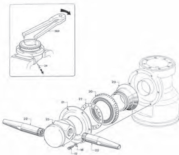
Gear subassembly
