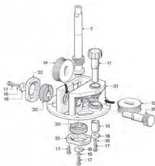
Gear subassembly
