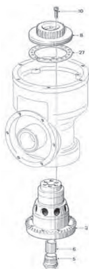
Stem subassembly
